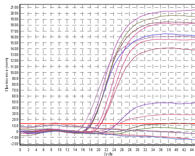
图3 A、B组免疫后28天荧光PCR检测曲线
