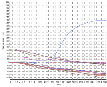
图2 A、B组免疫前荧光PCR检测曲线
